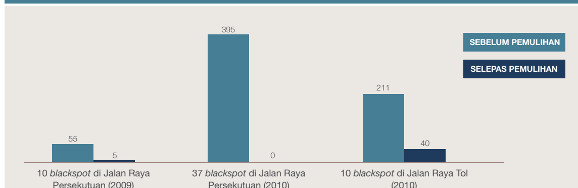
Rajah 1: Statistik Kemalangan Sebelum dan Selepas Pemulihan Blackspot Kemalangan Jalan Raya
